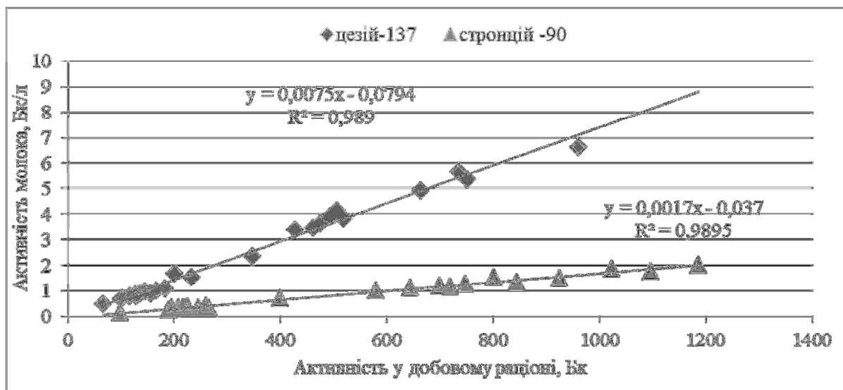
Рис. 1. Залежність між активністю ^{137}\text{Cs} і ^{90}\text{Sr} у добовому раціоні корів та молоці
